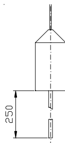
Pos. 24 Stachel für Fühlgewicht
